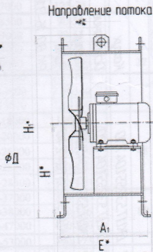
Вентиляторы ВО 14-320
