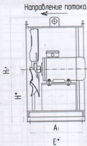
Вентиляторы ВО 06-300
